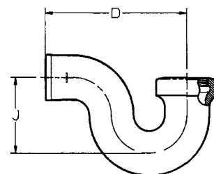
TAP P-TRAP
