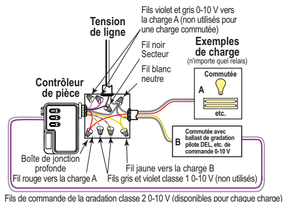
Connexions de classe 2 0-10 V
