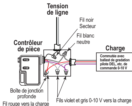
LMRC-111 avec gradation de classe 1
