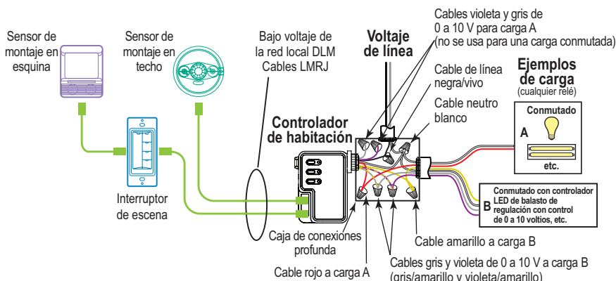
LMRC-111 con atenuación Clase 1
