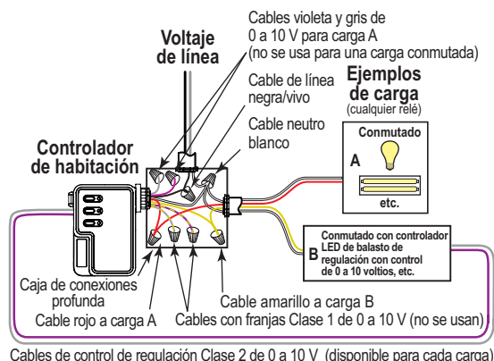
Conexiones Clase 2 de 0 a 10 V
