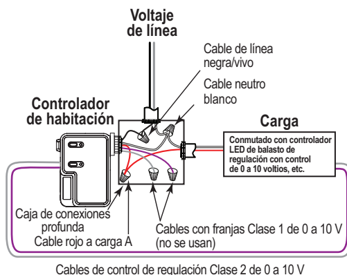
LMRC-111 con atenuación Clase 2
