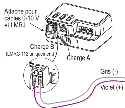
Connexions de classe 2 0-10 V
