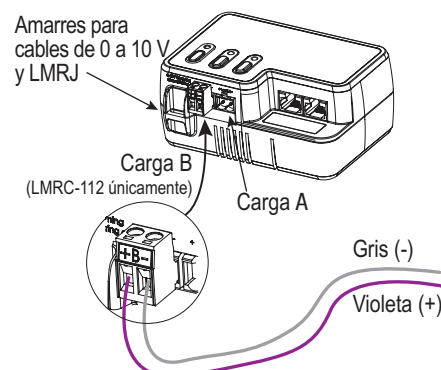
Conexiones Clase 2 de 0 a 10 V
