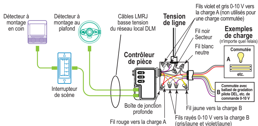
LMRC-111 avec gradation de classe 1
