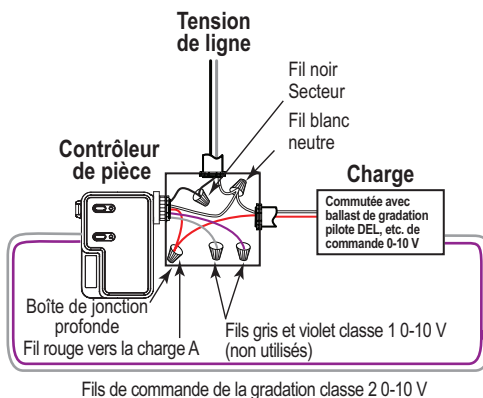
LMRC-111 avec gradation de classe 2
