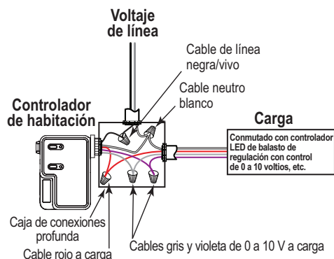
LMRC-111 con atenuación Clase 1
