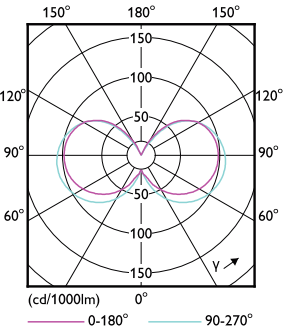
LEDbulb ST19 8,8W E26 950 CL
