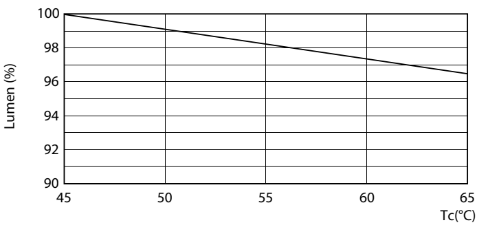
LEDtube FA8 4000K 240D LumenVsTc
