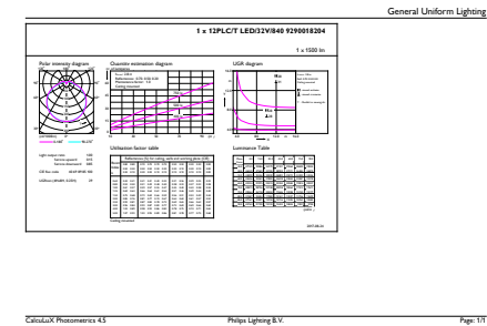
LEDtube PLC/T 12W G24Q 840 32V DIM
