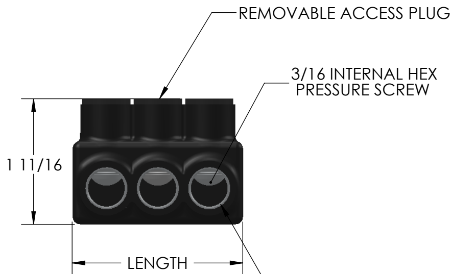
IPL1/0-3 SHOWN
