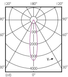
10-75W E26 PAR30L 25D 827 2700K
