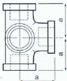
Side Outlet Tee
