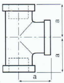
Tee
