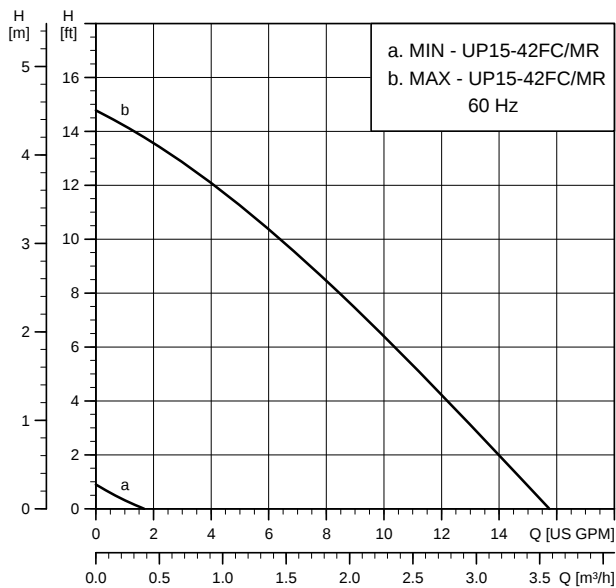
UP 15-42 FC/MR
