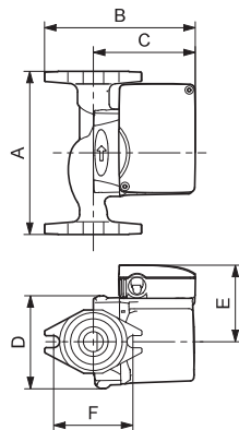
UP 15-42 FR
