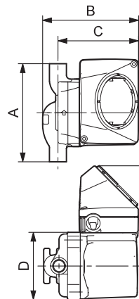
UP 15-10 B5/TLC
