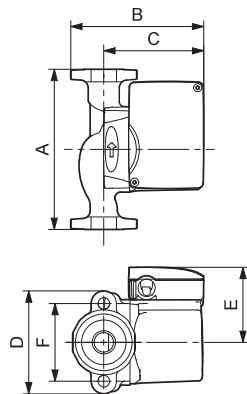
UP 15-42 F
