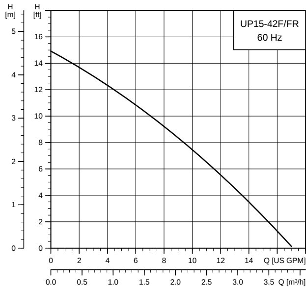
UP 15-42 F
