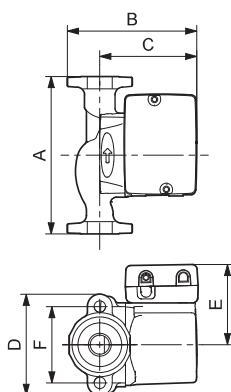
UP 15-42 F/VS
