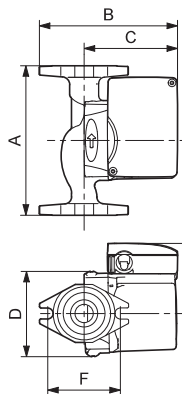
UP 15-10 FR
