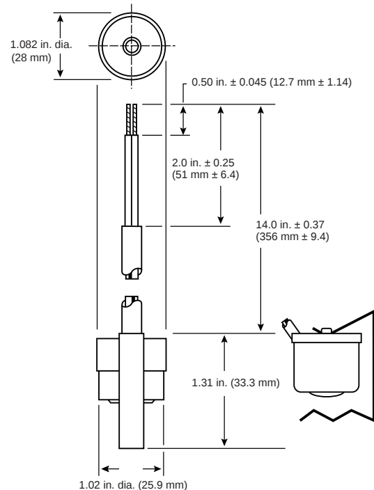
Fig. 14 AquaStat dimensions
