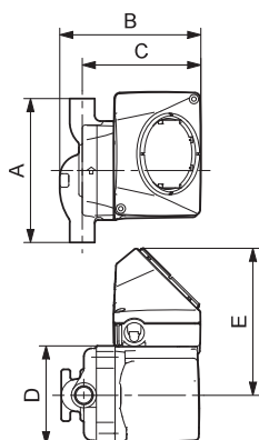
UP 15-42 B5/TLC
