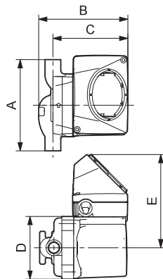
UP 15-18 B5/TLC
