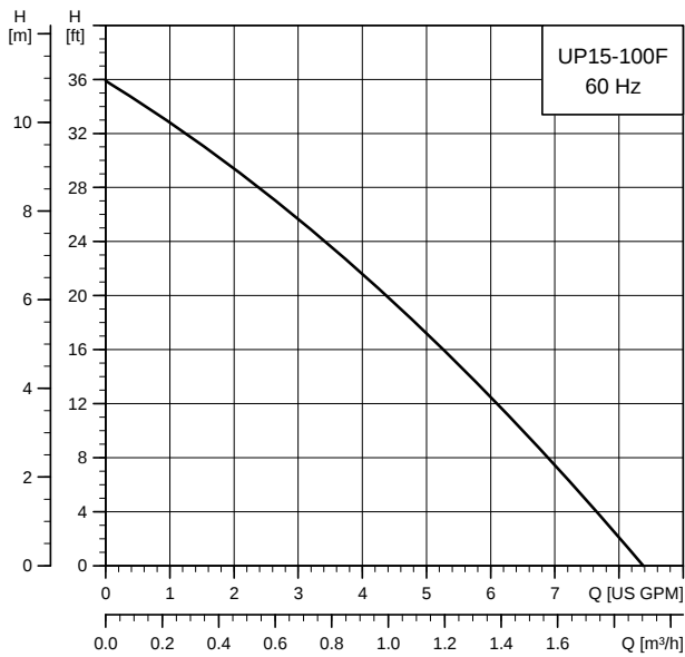
UP 15-100 F
