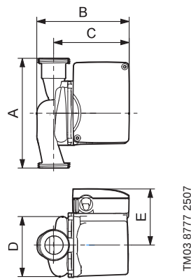
UP 15-29 SU
