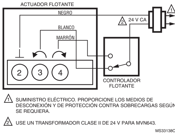
Fig. 17. MVN613 o MVN643 con control de dos posiciones.
