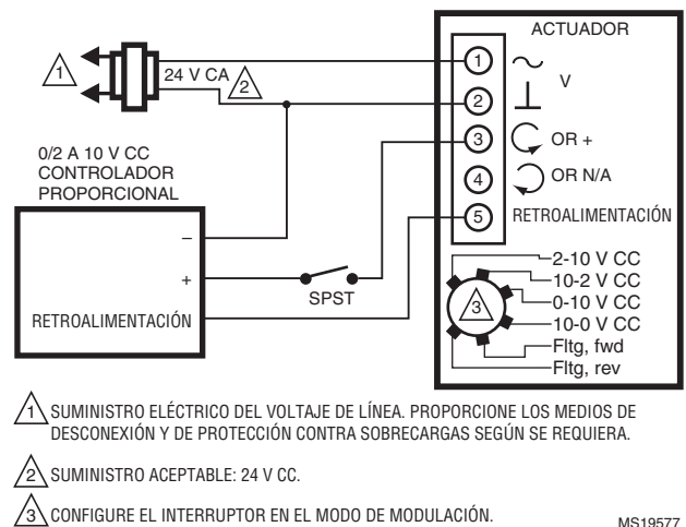
Fig. 13. MS7505 con control de sobrecomando para la posición completamente cerrada (configuración del modo de modulación).
