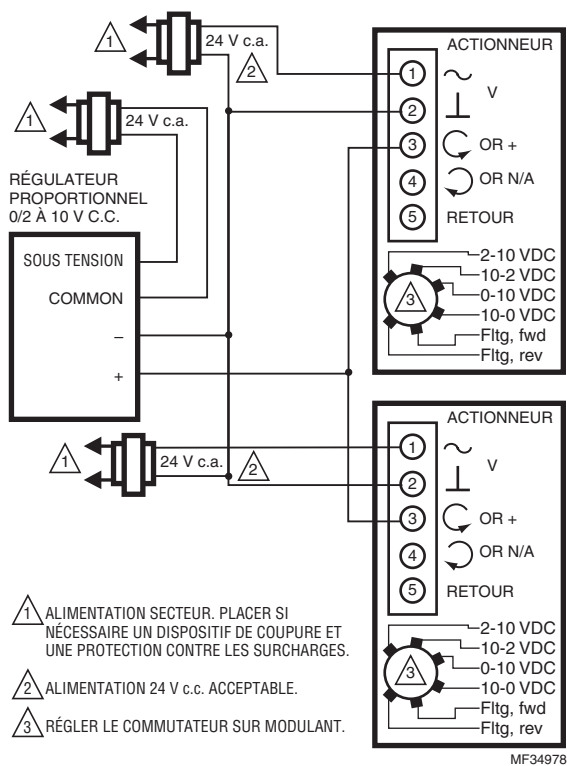
Fig. 15. MS7505 avec régulateurs proportionnels actionnant plusieurs actionneurs (réglage en mode modulant).
