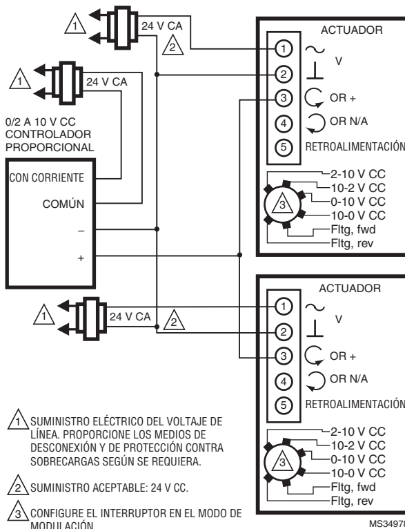
Fig. 15. MS7505 con controladores proporcionales que hacen funcionar múltiples actuadores (configuración del modo de modulación).
