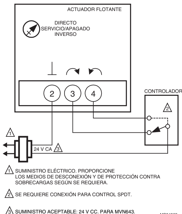
Fig. 7. MN6105 con control On/Off (encendido/apagado).
