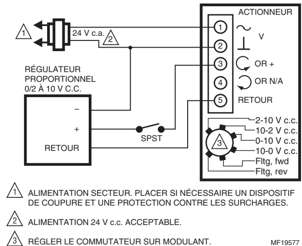
Fig. 13. MS7505 avec dérivation pour fermeture complète (réglage en mode modulant).
