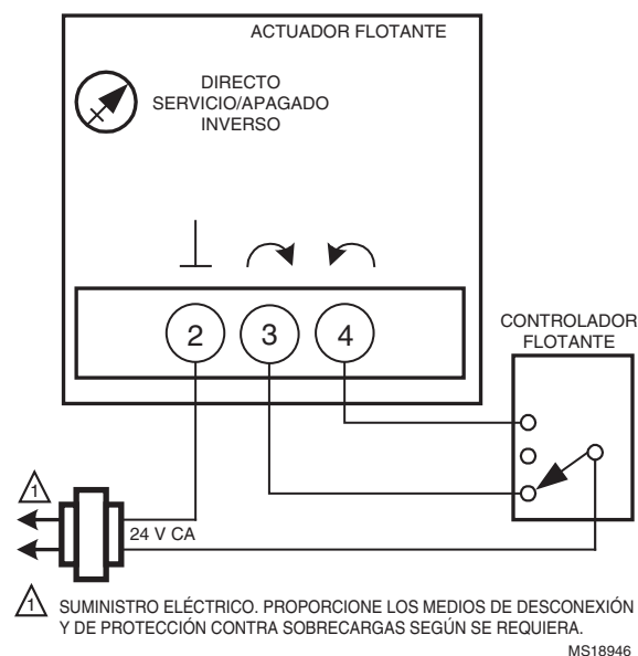
Fig. 8. MN6105 con control flotante.
