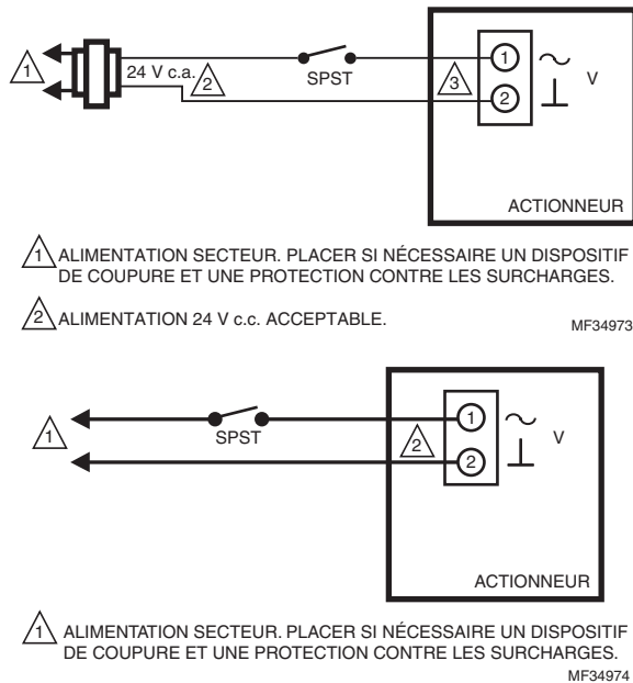
Fig. 10. MS8105 pour action Marche/Arrêt.
