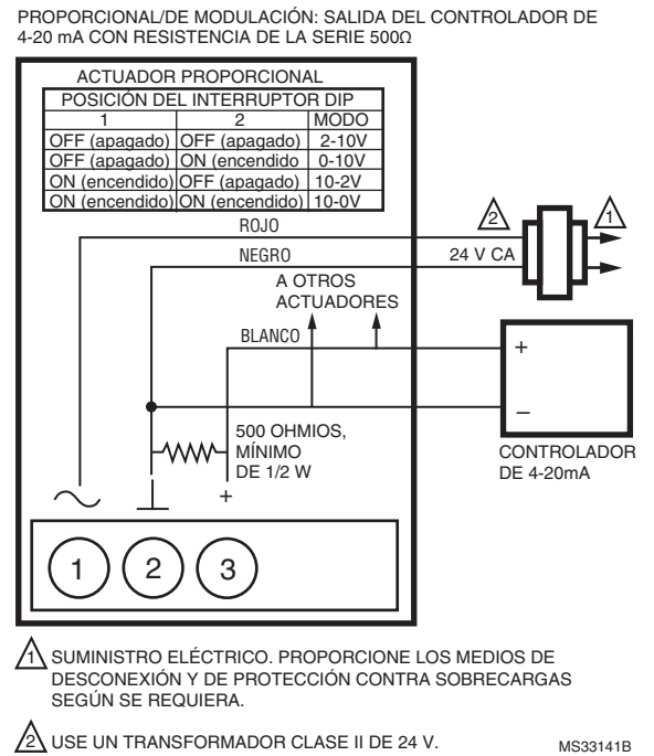
Fig. 19. MVN713 con control de 4-20 mA.
