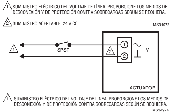
Fig. 10. MS8105 con control On/Off (encendido/apagado).
