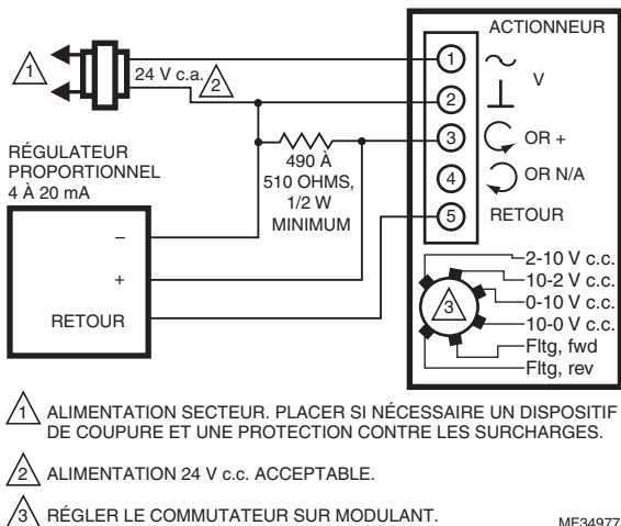
Fig. 14. MS7505 avec régulateurs proportionnels (réglage en mode modulant).
