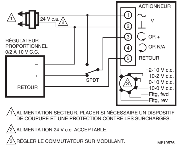
Fig. 12. MS7505 avec dérivation pour ouverture complète (réglage en mode modulant).
