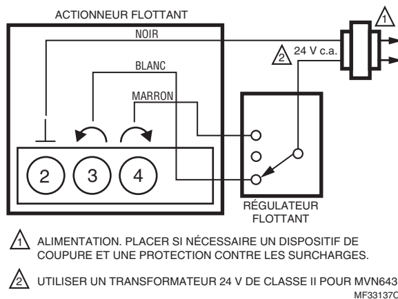
Fig. 16. MVN613 ou MVN643 avec commande flottante
