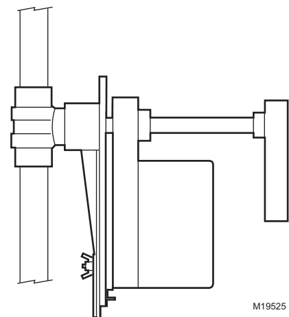
Fig. 4. Installation verticale du clapet.
