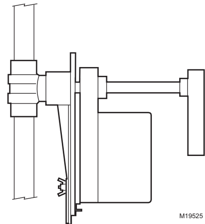
Fig. 4. Instalación vertical de la válvula.
