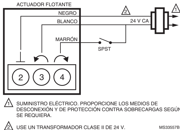
Fig. 18. MVN643 con control SPST de dos posiciones.
