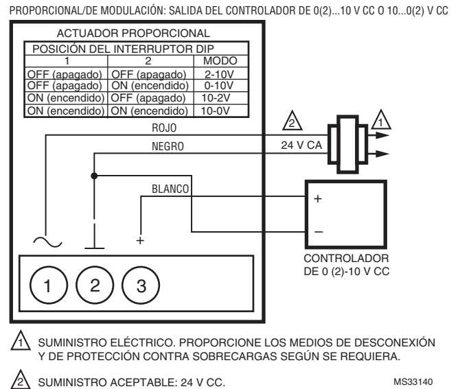
Fig. 20. MVN713 con control de 0 (2)-10 V CC.
