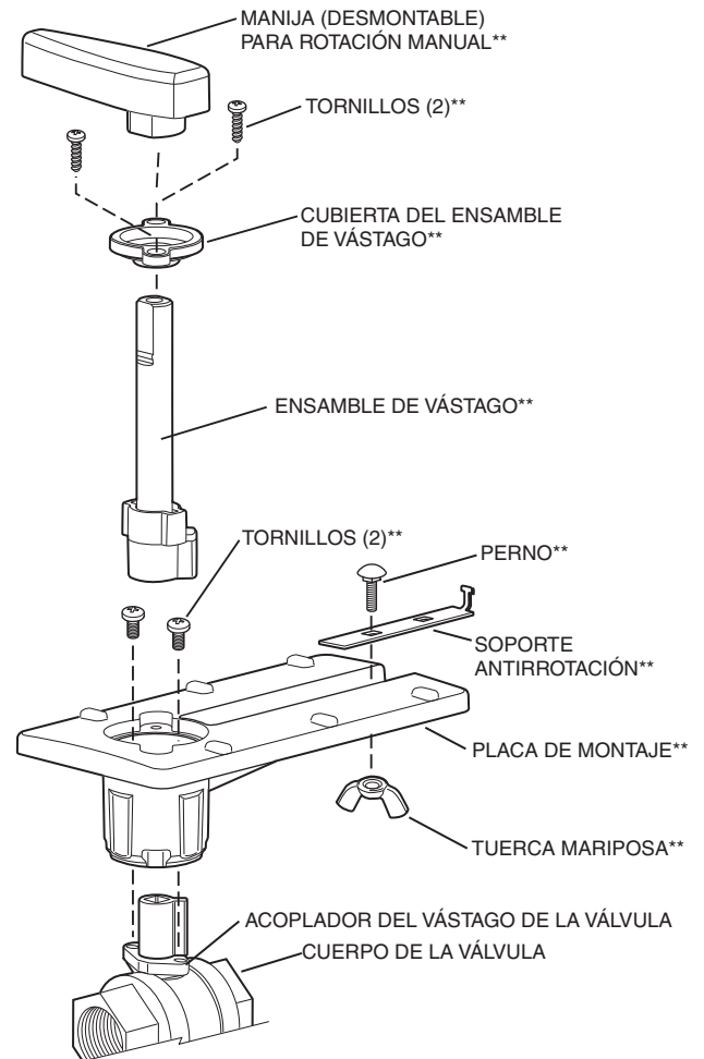
Fig. 3. Vista en despiece del ensamblaje de la válvula.
