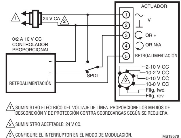
Fig. 12. MS7505 con control de sobrecomando para la posición completamente abierta (configuración del modo de modulación).
