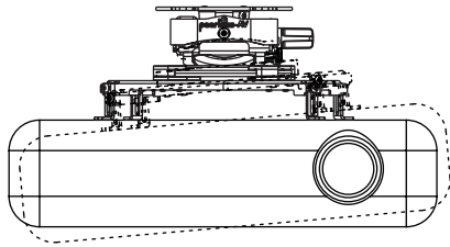
+/- 5° ROLL
