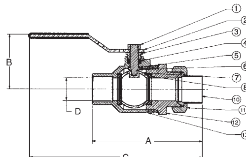
S-585-70-66-SU C x C
